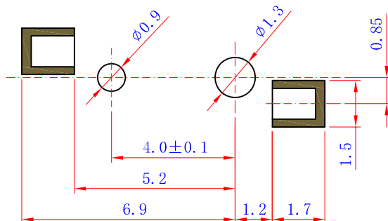
安装尺寸图
