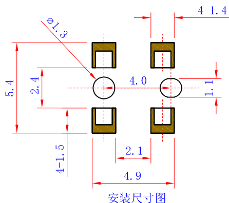
安装尺寸图
