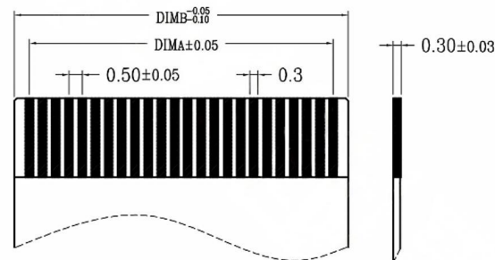
适用扁平线
